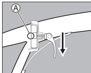
③レバーペダル部を垂直に下げ、折りたたみロックを固定します。 ※クイックレバーは必ずきつくしめてください。※きつくしない場合はAのネジをしめて調整してください。
