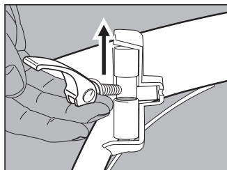
②クイックレバーを自転車後方へ水平に回転させ中央付近でレバーを上へ持ち上げ、前フレームと後フレームのロックを解除します。
